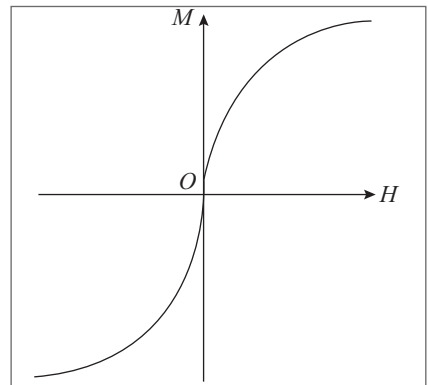
Figura 11.10 Curva de magnetização de um material ferromagnético.
