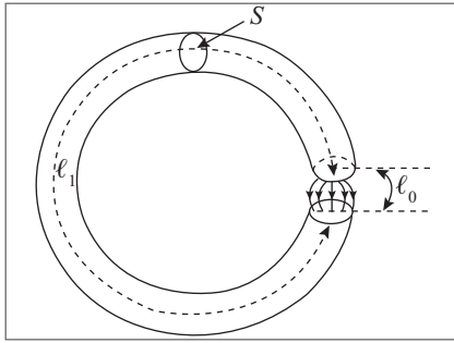
Figura 11.16 Entreferro.
