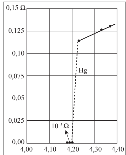
Figura 6.13 Resistência de Hg \times temperatura (em K).
