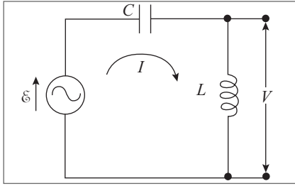
Figura 10.31 Circuito bloquador de baixas frequências.
