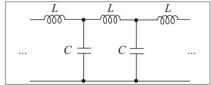
Figura 10.34 Filtro transmissor de baixas frequências.
