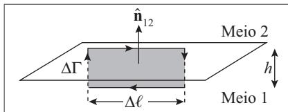
Figura 5.18 Circuito \Delta\Gamma .
