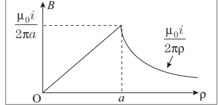
Figura 8.5 Magnitude de \mathbf{B} em função da distância ao eixo.
