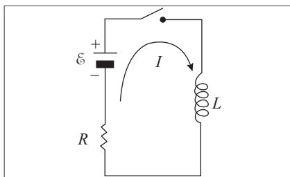
Figura 10.10 Circuito R-L.
