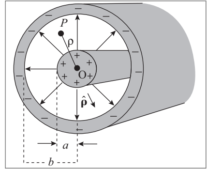
Figura 5.2 Capacitor cilíndrico.
