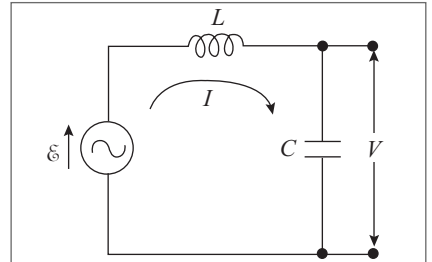
Figura 10.30 Circuito bloqueador de altas frequências.
