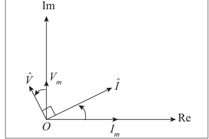
Figura 10.17 Representação complexa de \hat{V} e \hat{I} para um indutor.
