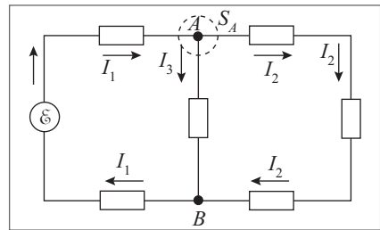
Figura 10.6 Circuito com duas malhas.
