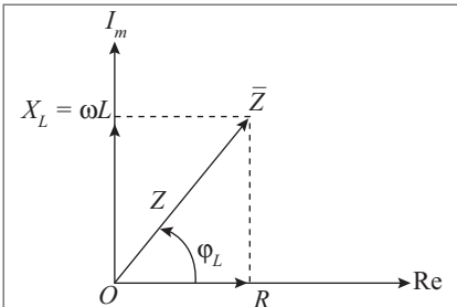
Figura 10.21 Impedância complexa do circuito R - L .
