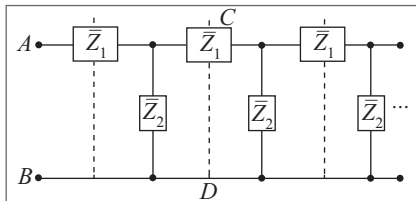
Figura 10.33 Redivisão de filtro infinito.
