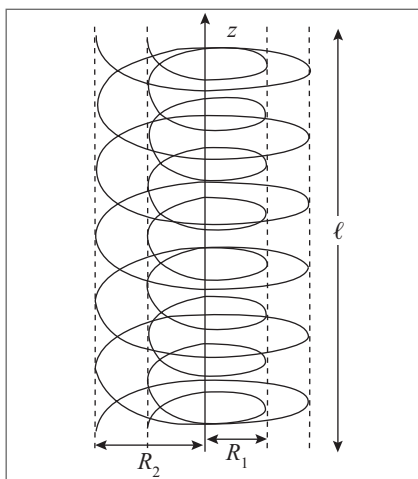
Figura 9.15 Indutância mútua entre dois solenoides.
