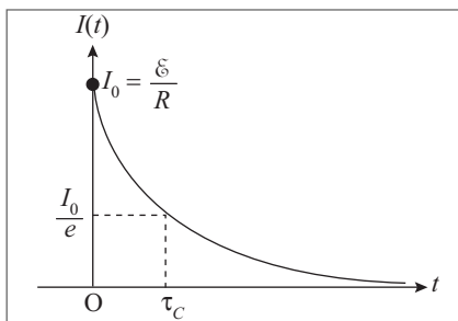
Figura 10.9 Corrente de carga de um capacitor.
