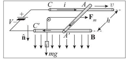
Figura 9.8 Modelo de motor linear.
