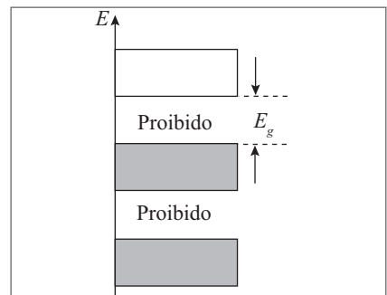
Figura 6.11 Bandas de energia num isolante.
