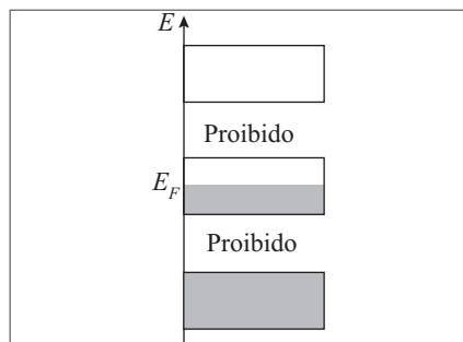
Figura 6.12 Bandas de energia num metal.
