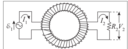
Figura 10.28 Bobinas toroidais acopladas.
