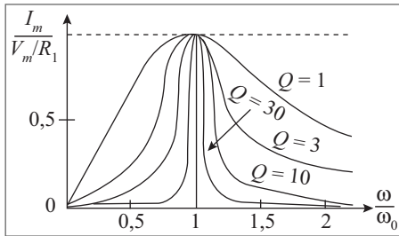
Figura 10.26 Curvas de ressonância para a amplitude.
