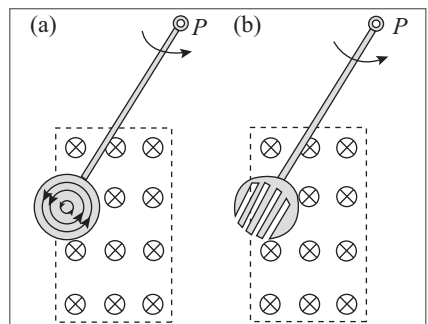
Figura 9.6 Corrente de Foucault.
