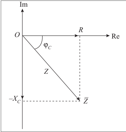
Figura 10.23 Impedância complexa do circuito R-C.
