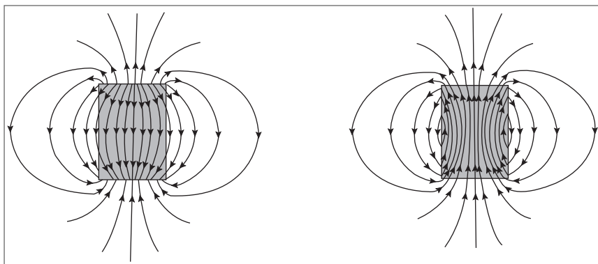
Figura 11.19 Linhas de \mathbf{H} (à esquerda) e de \mathbf{B} (à direita) num ímã permanente.
