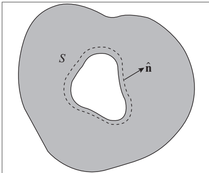
Figura 4.23 Condutor oco e superfície gaussiana S .
