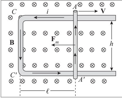
Figura 9.7 Haste metálica móvel sobre trilhos num campo B .
