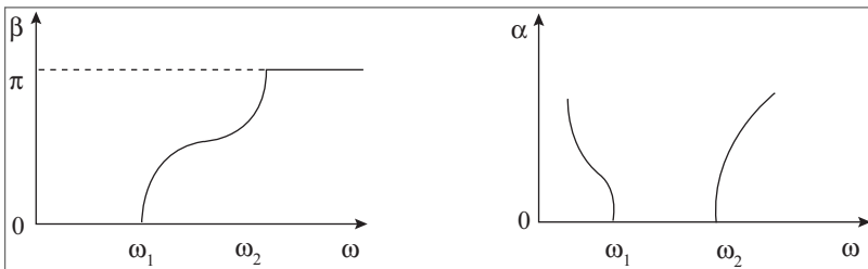
Figura 10.37 Comportamento de \beta e \alpha para o filtro transmissor de banda.
