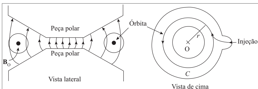
Figura 9.13 Esquema de um bétatron.
