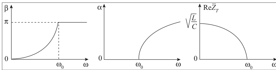
Figura 10.35 Gráficos de \beta , \alpha e \text{Re } \bar{Z}_T
