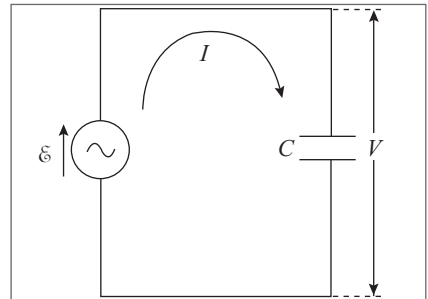
Figura 10.18 Capacitor e gerador AC.
