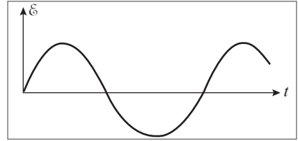
Figura 9.10 Força eletromotriz alternada.
