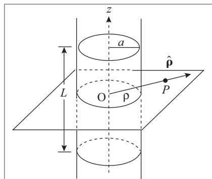
Figura 4.5 Cilindro circular condutor de raio a .
