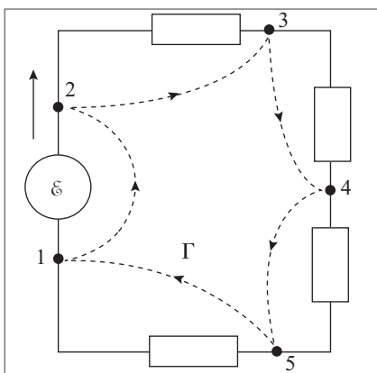
Figura 10.5 Circuito.
