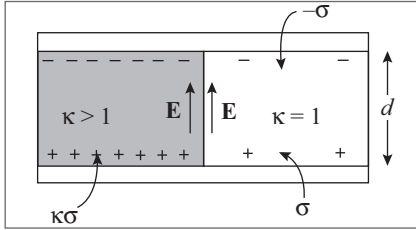
Figura 5.16 Capacitor semi-preenchido por dielétrico.
