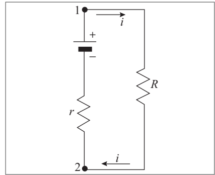
Figura 6.19 Circuito equivalente de uma bateria.
