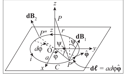
Figura 8.17 Campo de uma espira circular no eixo.
