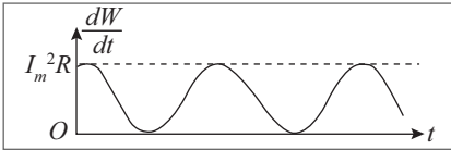
Figura 10.24 Potência instantânea AC dissipada em R.
