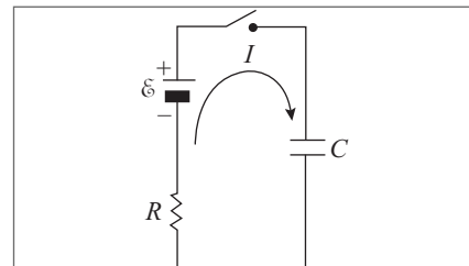
Figura 10.8 Circuito R-C.
