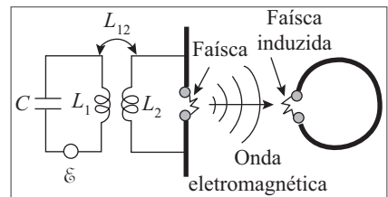
Figura 12.11 O experimento de Hertz.
