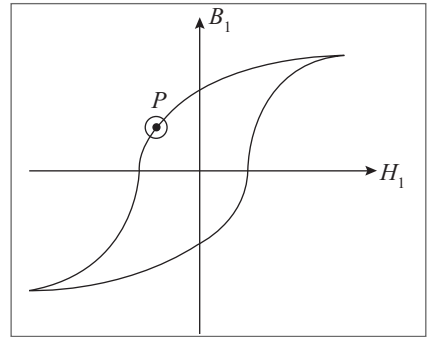
Figura 11.18 Ponto de operação P para ímã permanente.
