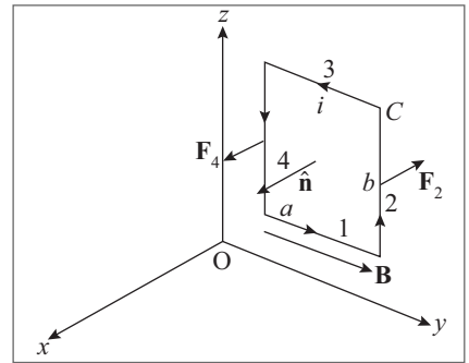
Figura 7.5 Espira retangular num campo \mathbf{B} uniforme.
