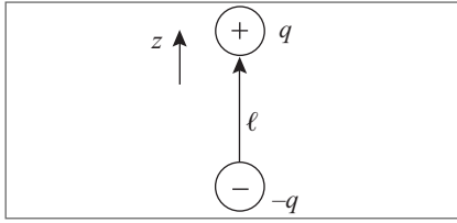
Figura 12.12 Dipolo hertziano oscilante.
