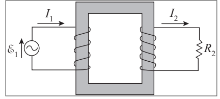
Figura 10.29 Transformador.
