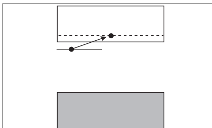
Figura 6.16 Impureza doadora.
