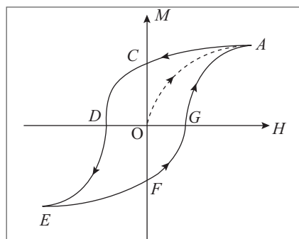
Figura 11.11 Ciclo de histerese.
