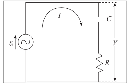
Figura 10.22 Circuito R - C com gerador A - C .
