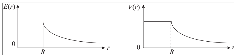
Figura 4.7 Campo radial E(r) e potencial V(r) para casca esférica ou esfera condutora.
