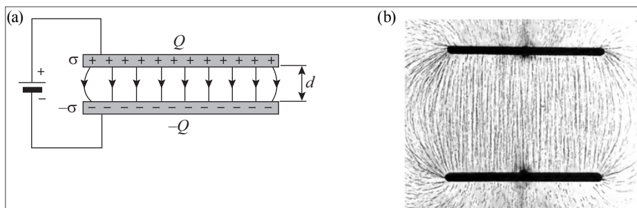
Figura 5.1 (a) Capacitor plano; (b) Linhas de campo elétrico observadas.
