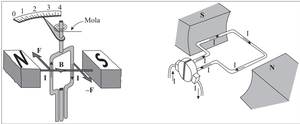
Figura 7.9 (a) Galvanômetro; (b) Motor de corrente contínua.
