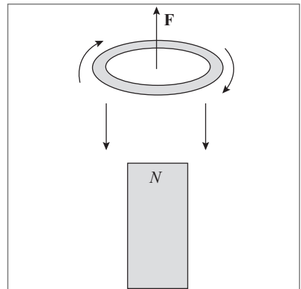
Figura 9.5 Espira condutora caindo sobre um ímã.
