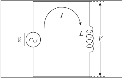
Figura 10.16 Indutor e gerador AC.
