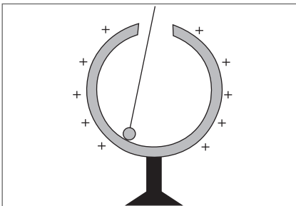
Figura 4.29 Experiência de Priestley.
