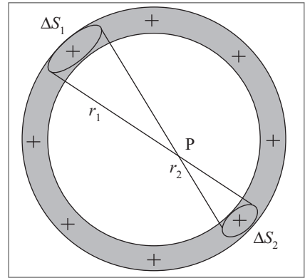
Figura 3.20 Cancelamento entre as contribuições de \Delta S_1 e \Delta S_2 .
