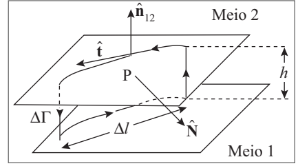
Figura 5.19 Vetores unitários na interface.
