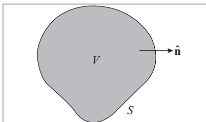
Figura 12.1 Teorema da divergência.
