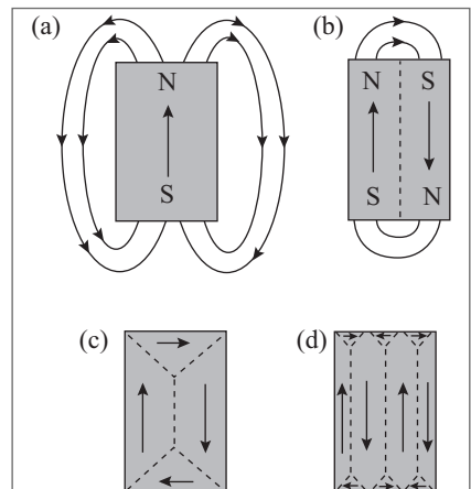
Figura 11.13 Domínios de Weiss.
