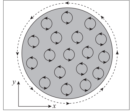
Figura 11.1 Correntes de Ampère num material magnético.
