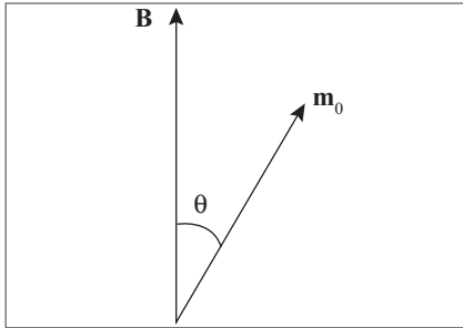
Figura 11.9 Dipolo magnético permanente no campo \mathbf{B} .
