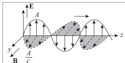
Figura 12.6 Onda plana monocromática.
