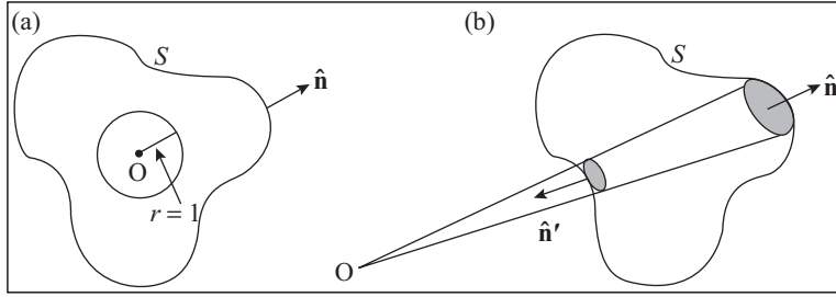
Figura 3.13 Ângulo sólido subtendido por uma superfície fechada S vista de um ponto O : (a) interno; (b) externo.
