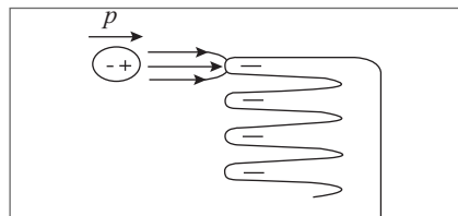
Figura 4.13 Atração de fragmento de papel por pente eletrizado.
