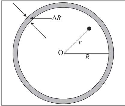
Figura 4.6 Casca esférica.
