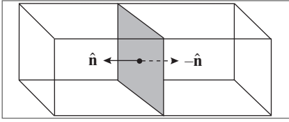
Figura 3.26 Fluxos sobre a face comum de elementos de volume adjacentes se cancelam.
