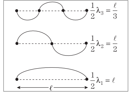
Figura 6.6 Modos de vibração.
