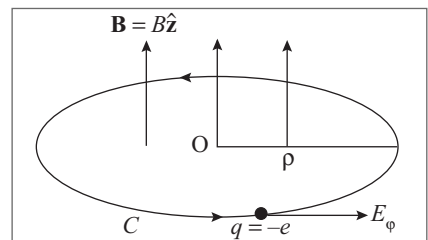
Figura 11.7 Coordenadas no átomo.
