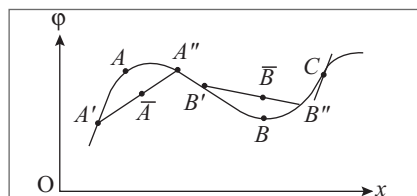
Figura 4.21 Curvatura e diferentes pontos de uma curva.
