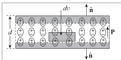
Figura 5.13 Polarização homogênea.
