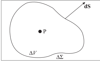
Figura 3.23 Volume \Delta V limitado por uma superfície \Delta\Sigma em torno de P.
