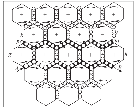
Figura 12.5 O modelo mecânico de Maxwell.
