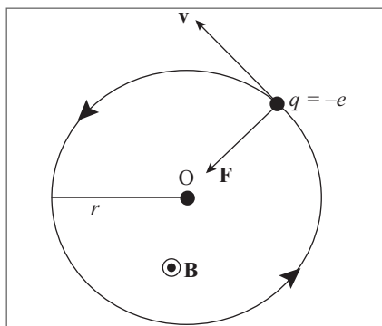
Figura 7.2 Órbita circular num campo \mathbf{B} ( \mathbf{B} aponta para cima).
