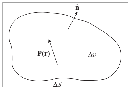
Figura 5.15 Volume dentro de um dielétrico.
