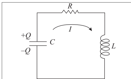
Figura 10.14 Circuito R-L-C.
