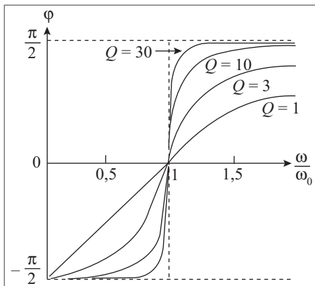
Figura 10.27 Curvas de ressonância para a fase.
