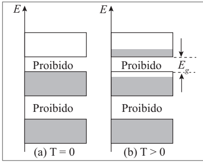
Figura 6.14 Espectro de bandas em semicondutores.
