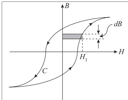
Figura 11.15 Ciclo de histerese e energia.
