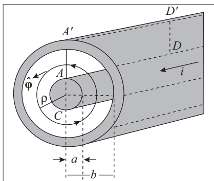
Figura 9.16 Cabo coaxial.
