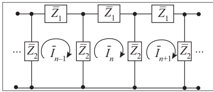
Figura 10.32 Filtro infinito.
