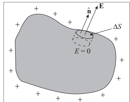
Figura 3.22 Superfície gaussiana (caixa cilíndrica) na superfície de um condutor.
