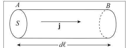
Figura 6.4 Trecho de fio condutor.
