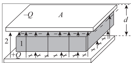
Figura 5.9 Capacitor plano com dielétrico.
