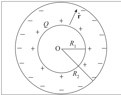
Figura 5.3 Capacitor esférico.
