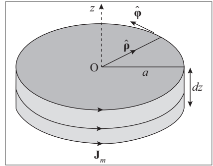
Figura 11.2 Corrente superficial no cilindro.
