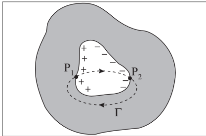
Figura 4.24 O circuito \Gamma .
