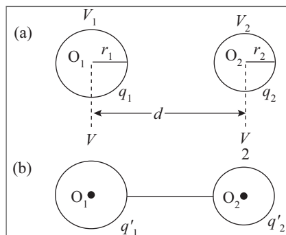
Figura 4.27 Esferas condutoras carregadas (a) isoladas; (b) ligadas.
