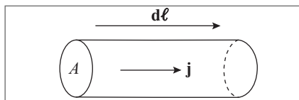
Figura 7.4 Trecho condutor com corrente \mathbf{j} .
