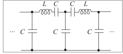
Figura 10.36 Filtro transmissor de banda.
