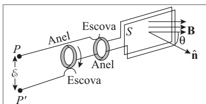
Figura 9.9 Modelo de gerador de corrente alternada.
