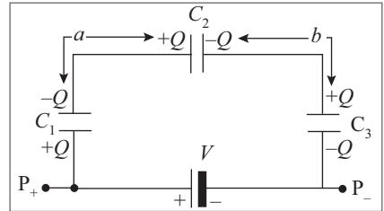
Figura 5.5 Conexão em série.
