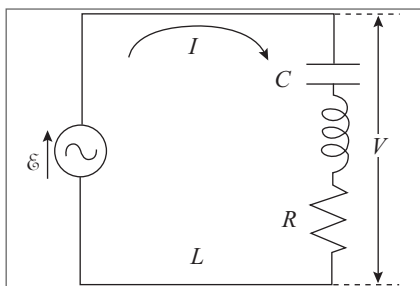
Figura 10.25 Circuito R - L - C com gerador AC.
