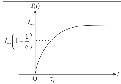
Figura 10.11 Crescimento da corrente no circuito R - L .
