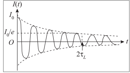
Figura 10.15 Oscilações amortecidas da corrente.
