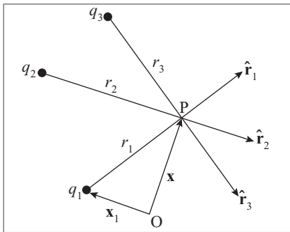
Figura 3.1 Campo de uma distribuição de cargas puntiformes num ponto P.
