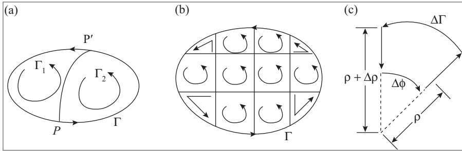
Figura 4.15 (a) Propriedade aditiva da circulação; (b) Decomposição de circuito em malhas; (c) Circuito \Delta\Gamma .
