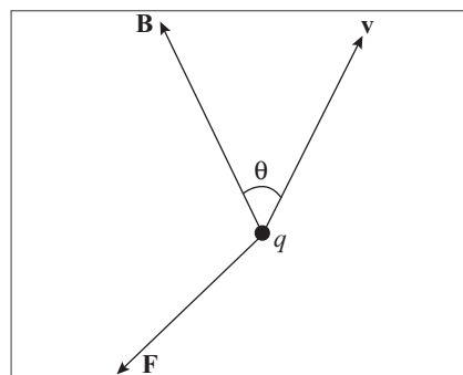
Figura 7.1 Força magnética sobre uma carga.
