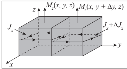
Figura 11.3 Magnetização inhomogênea: blocos adjacentes.
