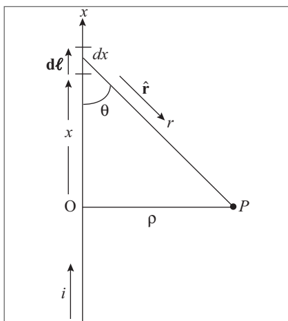
Figura 8.16 Fio retilíneo.
