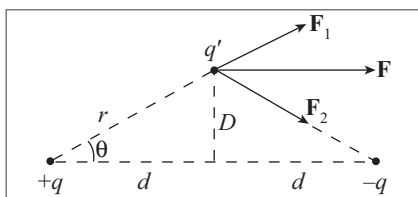
Figura 2.4 Forças sobre carga q' .
