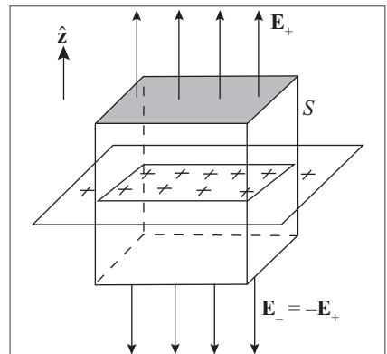
Figura 3.17 Superfície gaussiana S para um plano uniformemente carregado.
