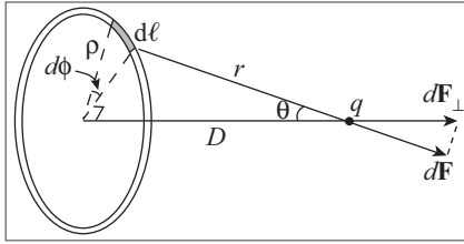
Figura 2.5 Força de um anel carregado sobre uma carga q .
