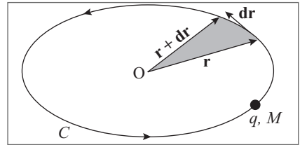
Figura 11.6 Órbita de Bohr.
