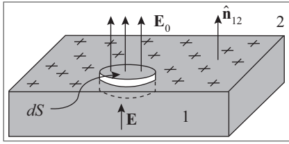
Figura 5.10 Superfície gaussiana.
