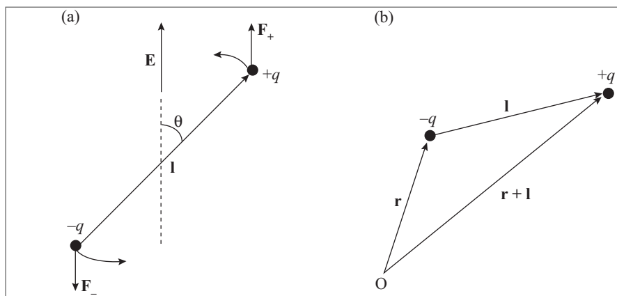
Figura 4.12 (a) Torque sobre um dipolo num campo uniforme; (b) Energia potencial de um dipolo num campo externo.
