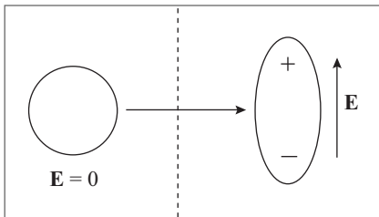
Figura 5.11 Criação de um dipolo.
