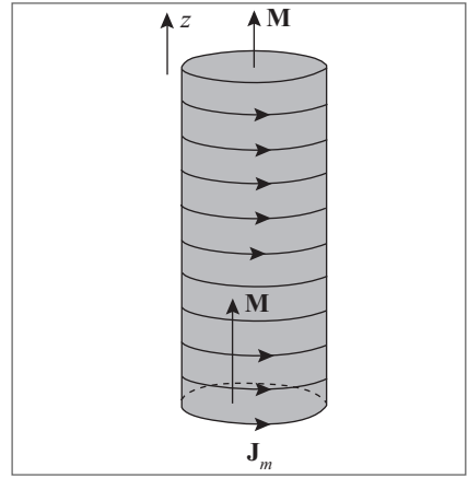
Figura 11.5 Cilindro homogeneamente magnetizado.
