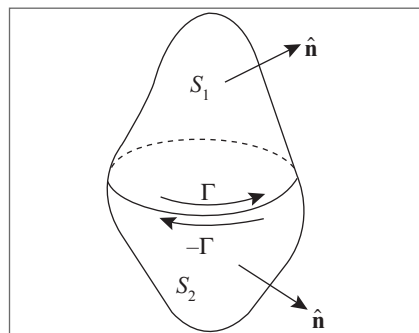
Figura 4.20 Superfície S_1 e S_2 de contorno comum \Gamma .
