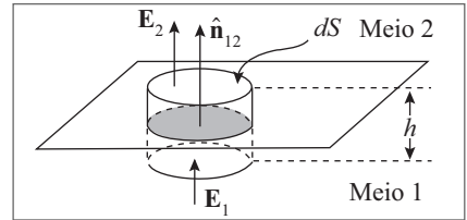
Figura 5.17 Superfície gaussiana.
