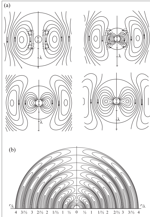
Figura 12.16 (a) Linhas de E (zona próxima); (b) Linhas de E (zona de onda).
