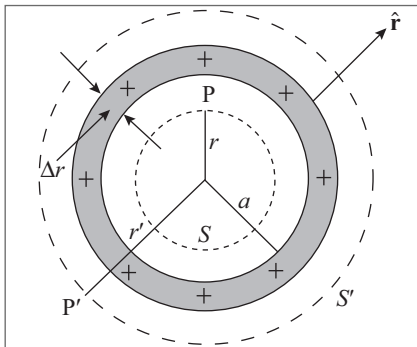
Figura 3.19 Camada esférica de carga e superfícies gaussianas S e S' .
