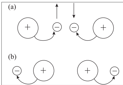
Figura 11.12 Ligação covalente (a) por elétrons de spins opostos.
