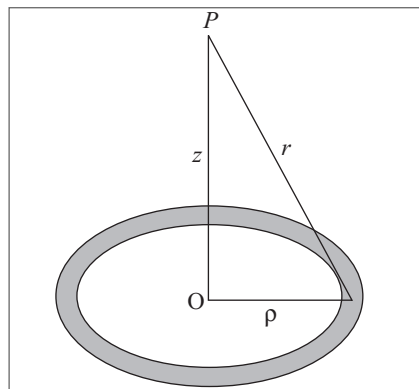
Figura 4.3 Anel carregado.
