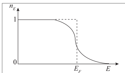
Figura 6.9 Distribuição de Fermi para T > 0 .
