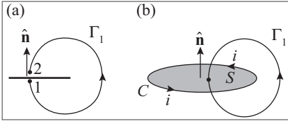
Figura 8.7 Circuito \Gamma_1 interrompido por uma barreira [(a) vista lateral].
