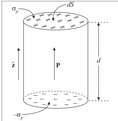
Figura 5.14 Cilindro polarizado.
