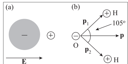
Figura 4.10 (a) Polarização da nuvem eletrônica no campo externo \mathbf{E} ; (b) Dipolo permanente da molécula de \text{H}_2\text{O} .
