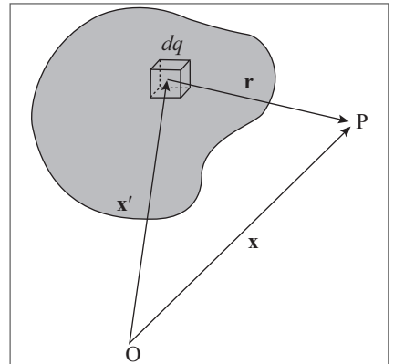
Figura 3.2 Campo de uma distribuição contínua de cargas num ponto P.
