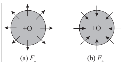
Figura 12.9 Os dois termos da (12.7.12).
