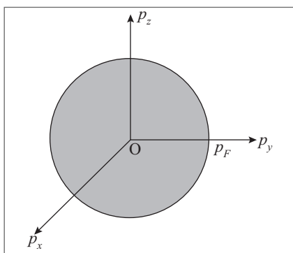
Figura 6.7 A esfera de Fermi.
