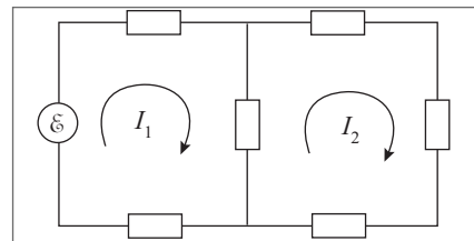
Figura 10.7 Correntes circulantes.
