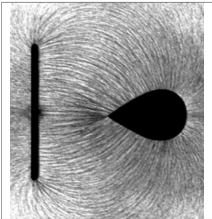
Figura 4.28 Poder das pontas.
