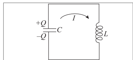
Figura 10.12 Circuito L - C .
