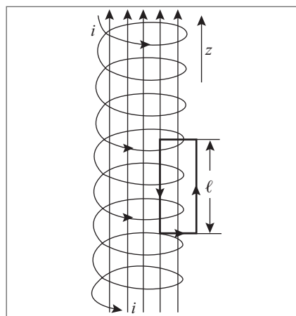
Figura 8.21 Solenoide.
